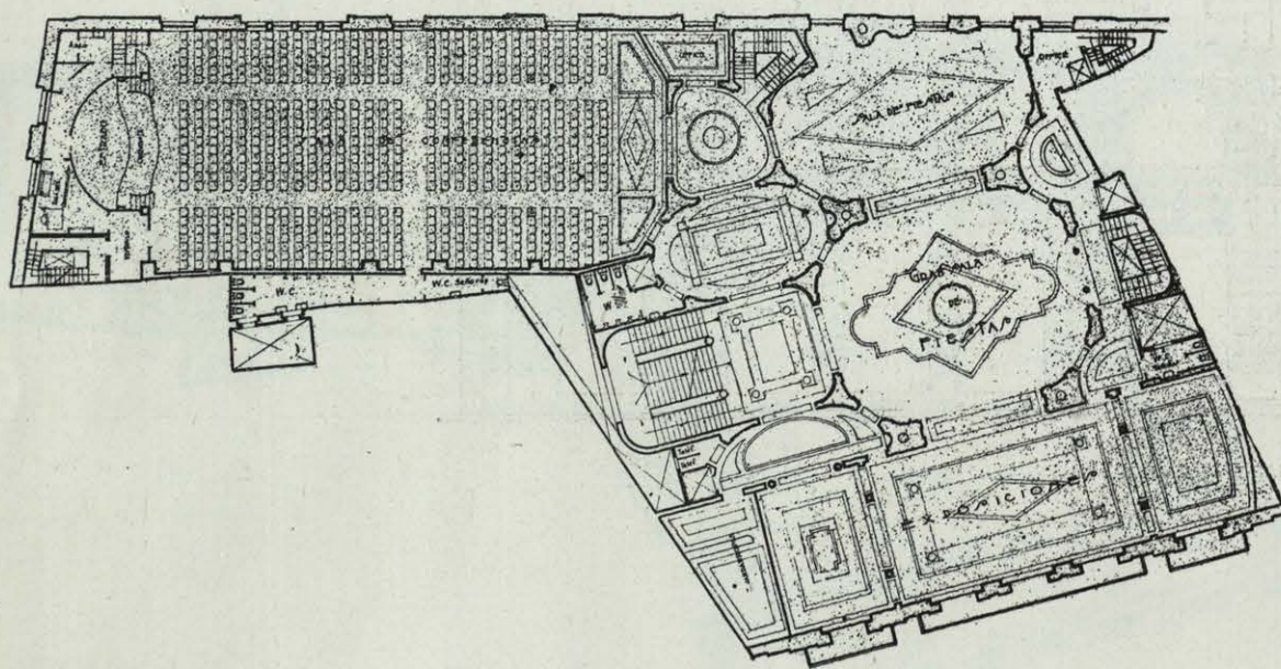
PLANTA PRINCIPAL.
