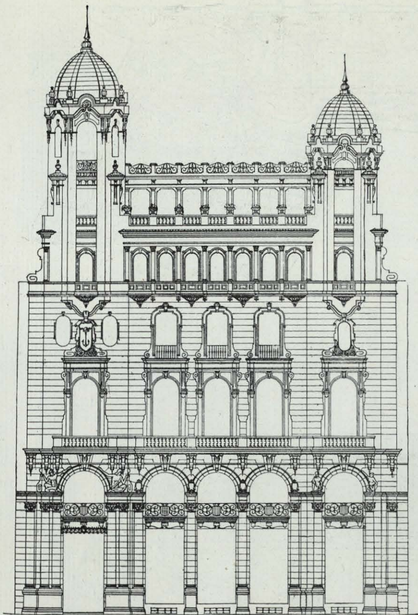
FACHADA PRINCIPAL.
